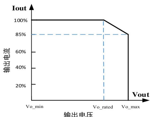
负载曲线
