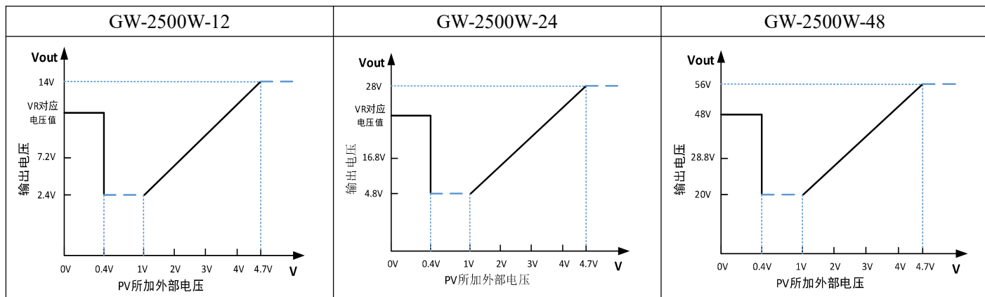
主路输出 PV 调压曲线
