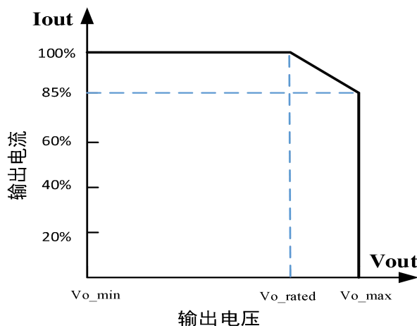
负载曲线
