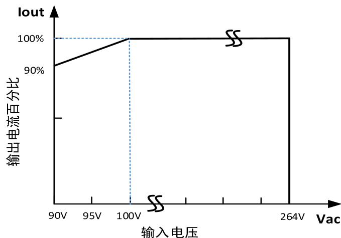
GW1600W-24V/48V 输出降额曲线
