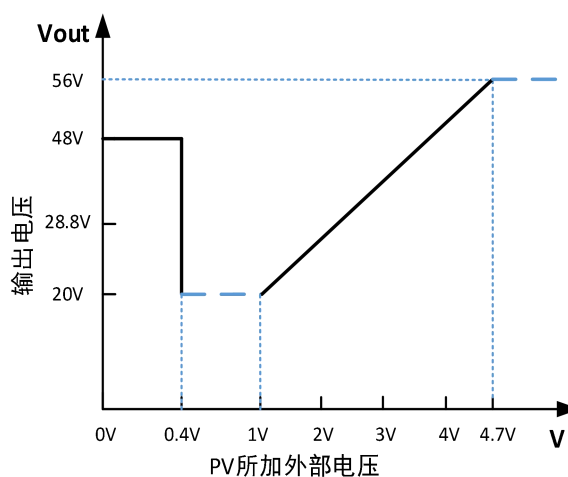
GW1600W-48 主路输出 PV 调压曲线
