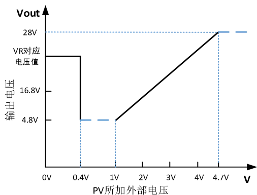
GW-3200W-24 主路输出 PV 调压曲线
