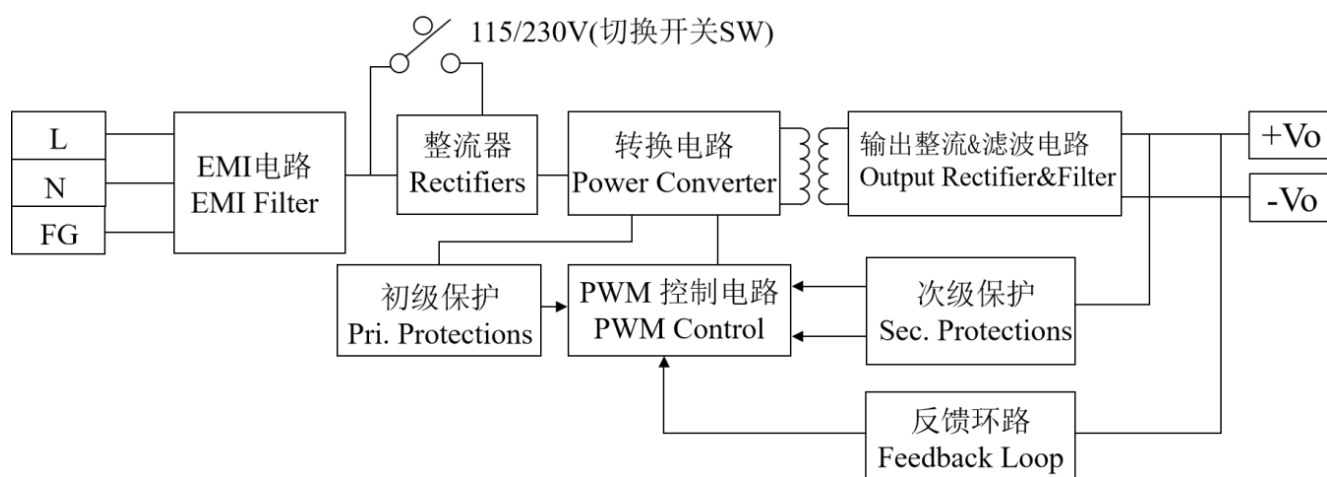
■ 方框图 Block Diagram
